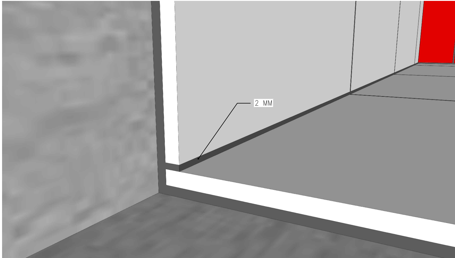
PERTEMUAN KERAMIK DINDING & LANTAI
