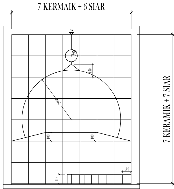
TAMPAK DEPAN
